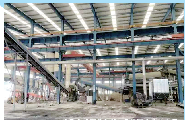
改造中的环龙智能工业机器人生产车间
